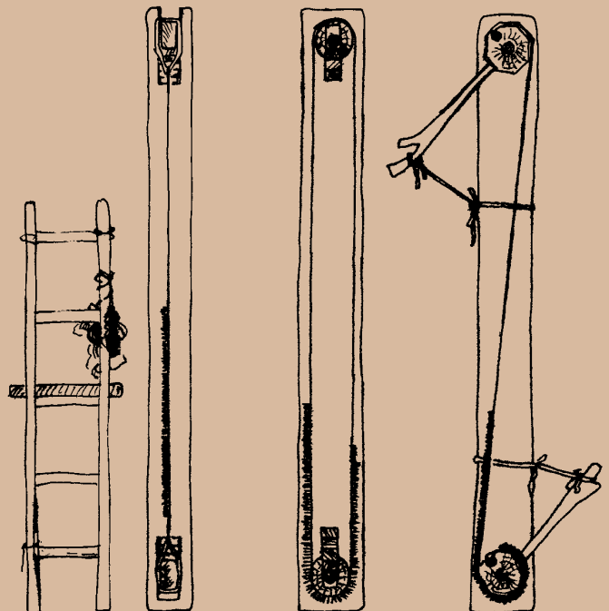
Kettfaden fixiert, Sitzbank in der Höhe verstellbar
